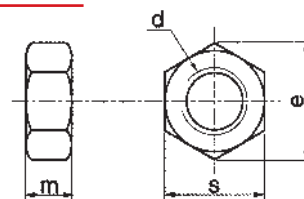
DIN 934 - A2 - A4
