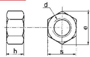
Hh - NFE 25-407 - A2 & A4
